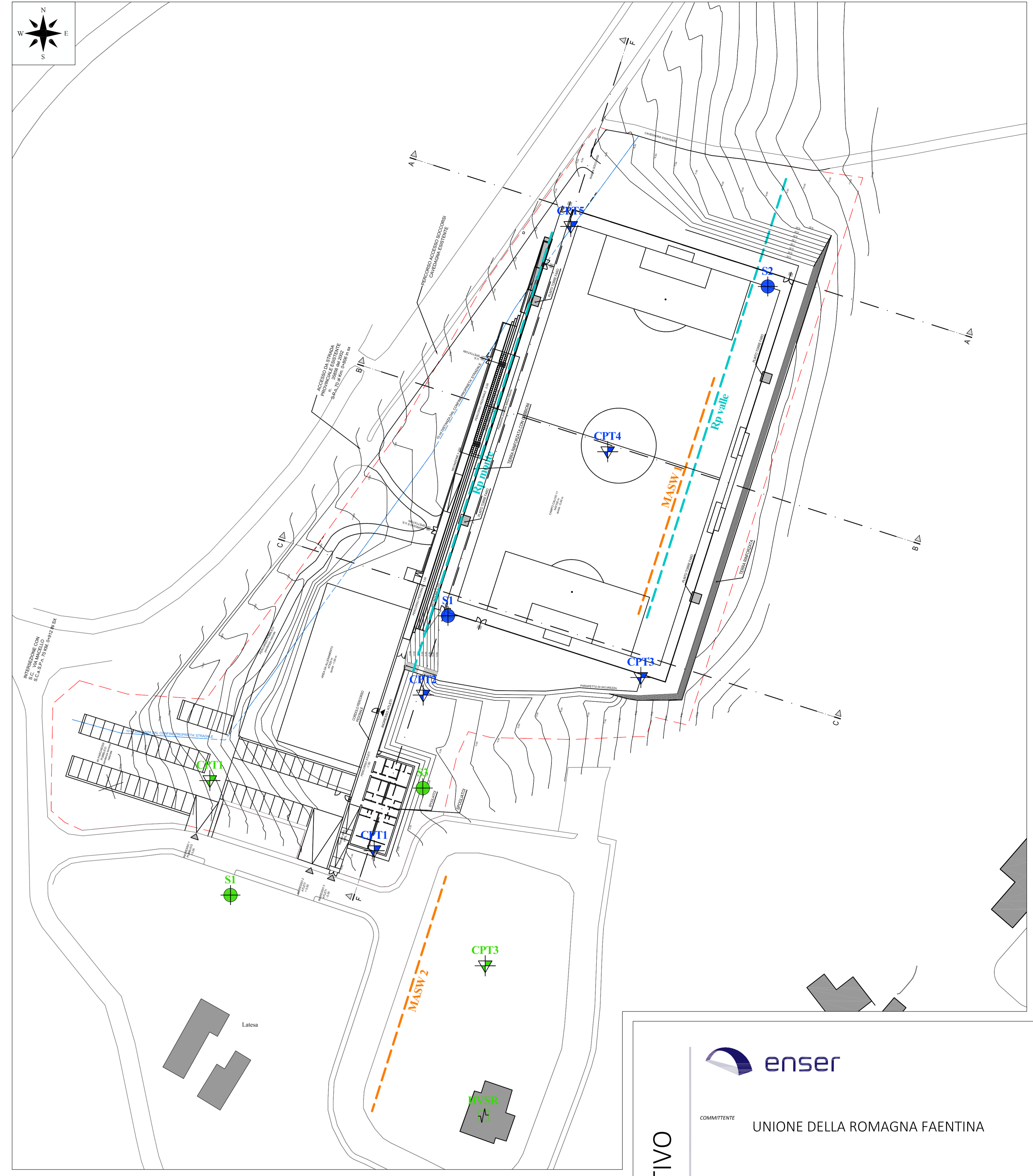
PLANIMETRIA GENERALE (scala 1:500)
